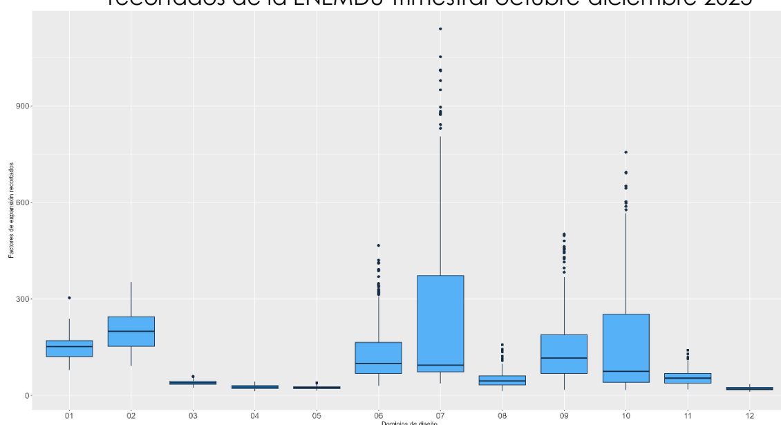
Gráfico 4. Diagramas de caja y bigote de los factores de expansión recortados de la ENEMDU Trimestral octubre-diciembre 2023
