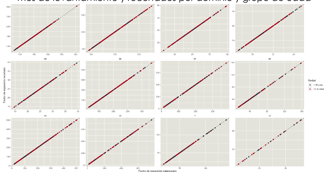
Gráfico 5. Comparación de los factores de expansión balanceados por mes de levantamiento y recortados por dominio y grupo de edad
