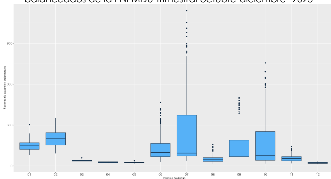
Gráfico 3. Diagramas de caja y bigote de los factores de expansión balanceados de la ENEMDU Trimestral octubre-diciembre 1 2023
