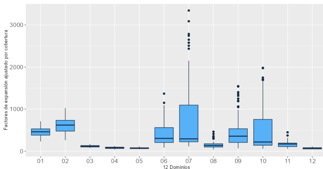
Gráfico 2. Diagramas de caja y bigote de los factores de expansión ajustados por cobertura de la ENEMDU abril 2024 1 .
