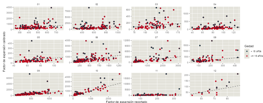
Gráfico 5. Comparación de los factores de expansión recortados y calibrados por dominio y grupo de edad.
