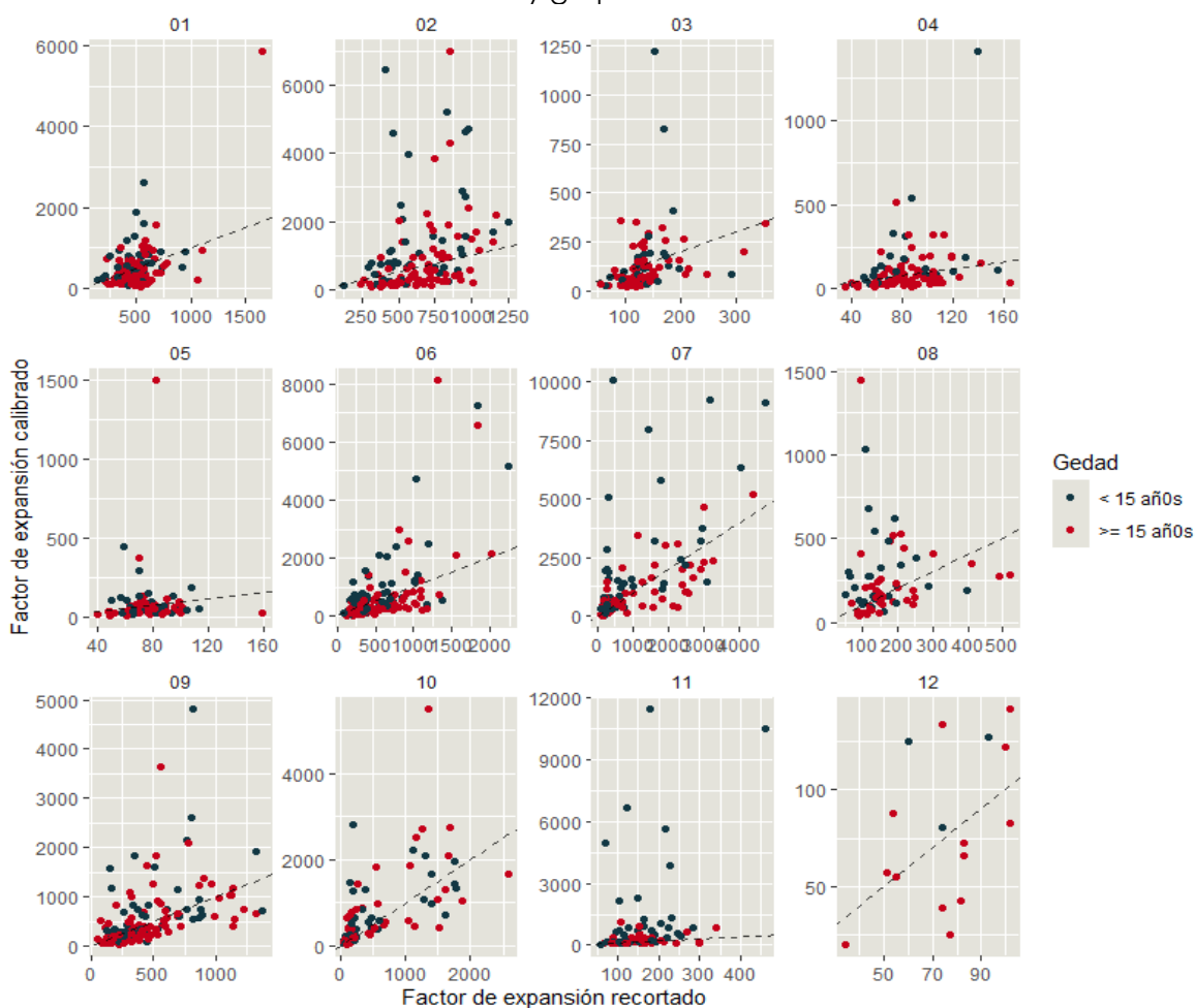
Gráfico 7 Comparación de los factores de expansión recortados y calibrados por dominio y grupo de edad.
