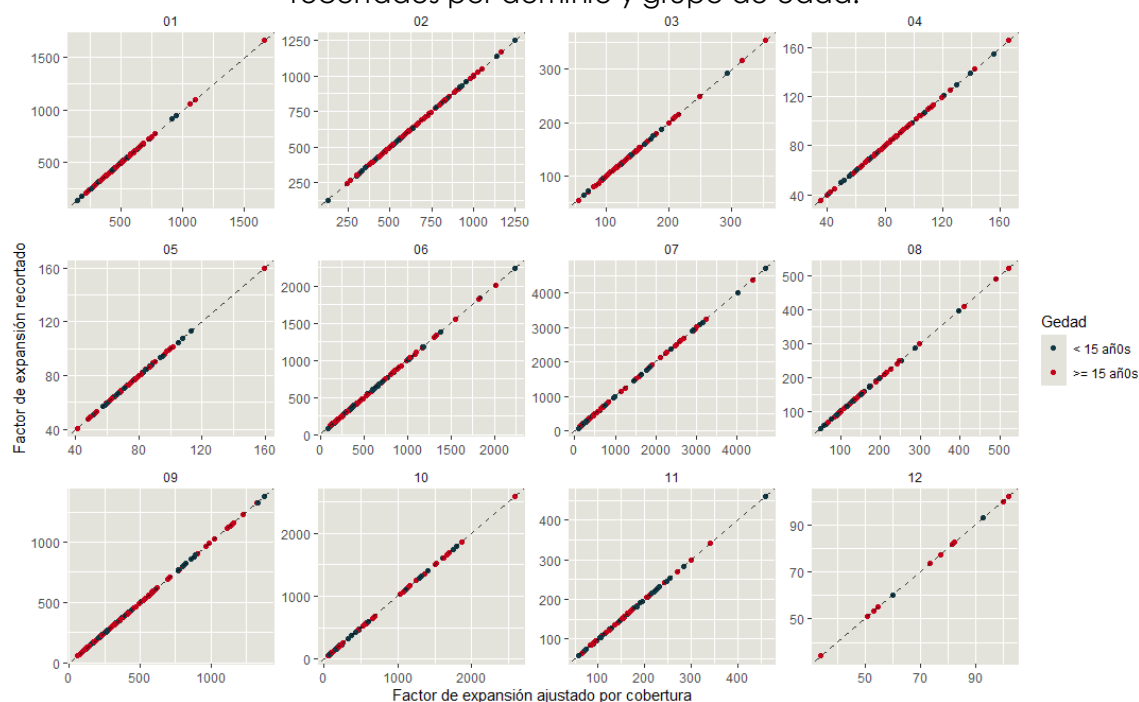
Gráfico 6 Comparación de los factores de expansión ajustados por cobertura y recortados por dominio y grupo de edad.
