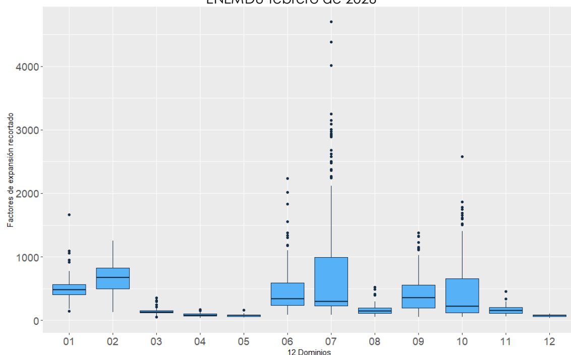
Gráfico 5 Diagramas de caja y bigote del factor de expansión recortados de la ENEMDU febrero de 2026
