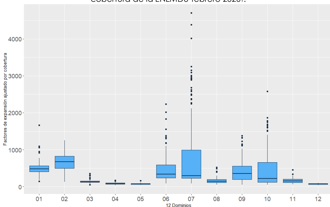
Gráfico 4 Diagramas de caja y bigote de los factores de expansión ajustados por cobertura de la ENEMDU febrero 2026 1 .
